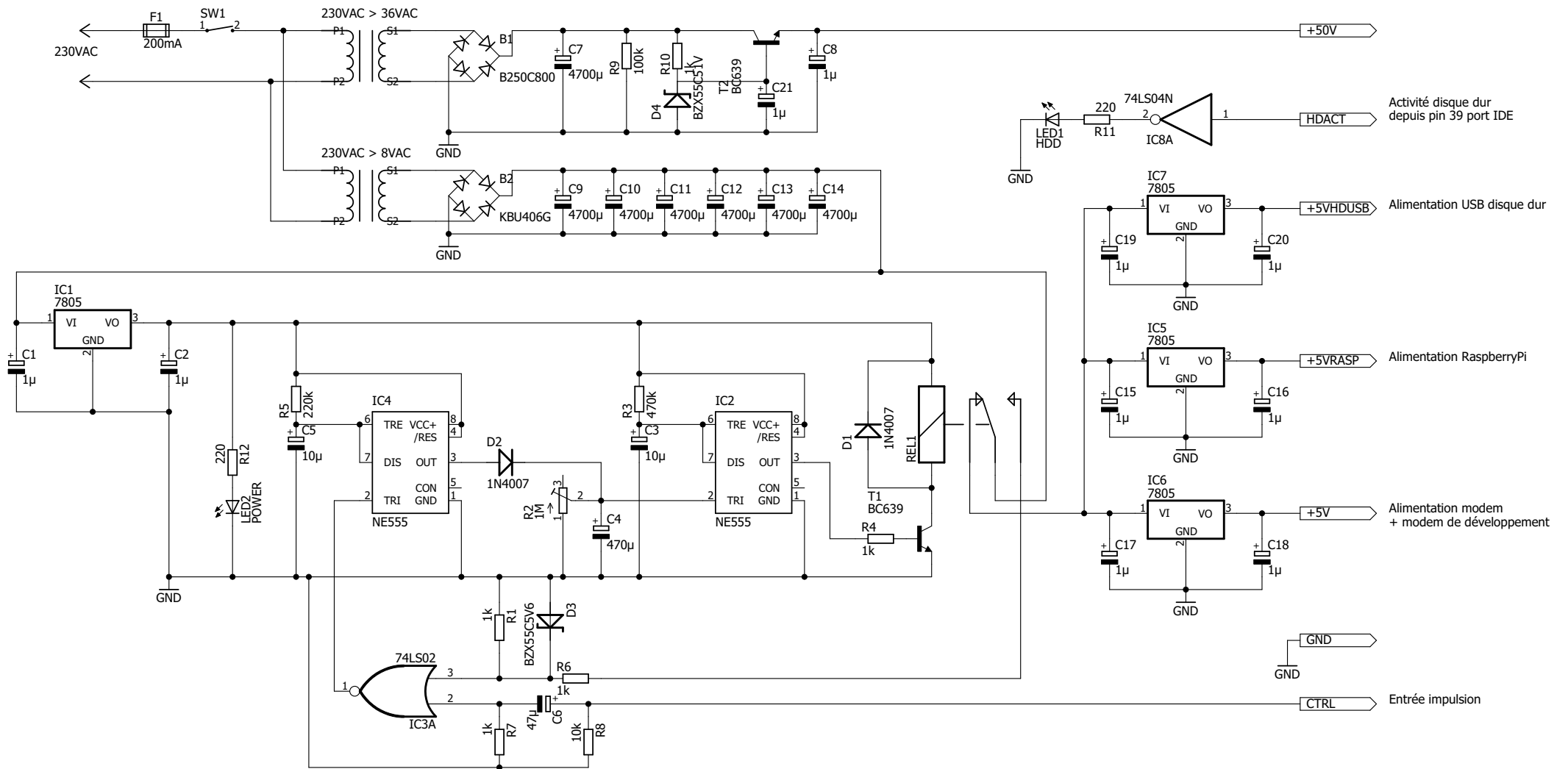
Serveur Minitel Alimentation avec reset automatique en cas de plantage de RaspberryPi Auteur: Jelora Date: 16/08/2017
